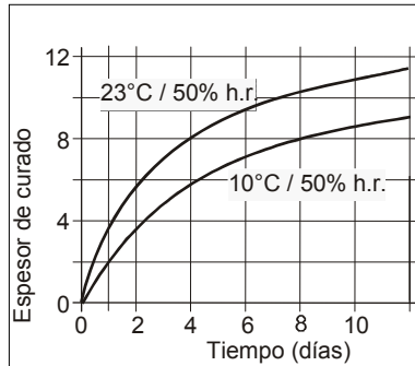
Diagrama 1: Velocidad de curado del Sikaflex®-221i
